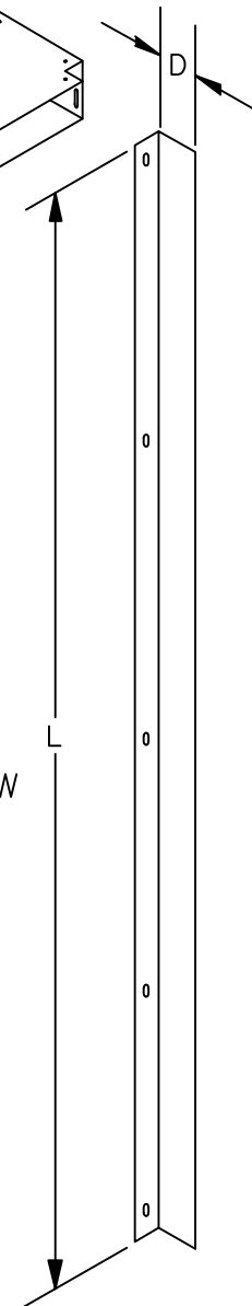
DIVIDER
